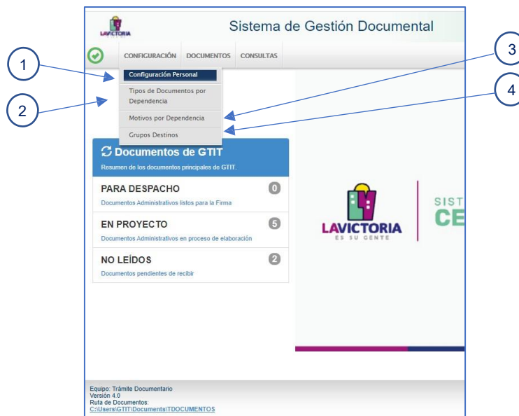
Figura 5. Menú configuración.
